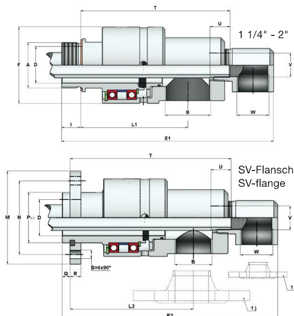
Maße für Innenrohr Dimensions syphon pipe
