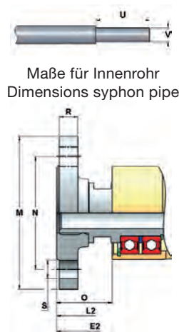
Schweißflansch Welded flange
