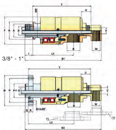
SV-Flansch SV-flange
